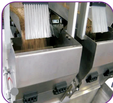
Canale vibrante, spazzola ferma prodotto e cestello
